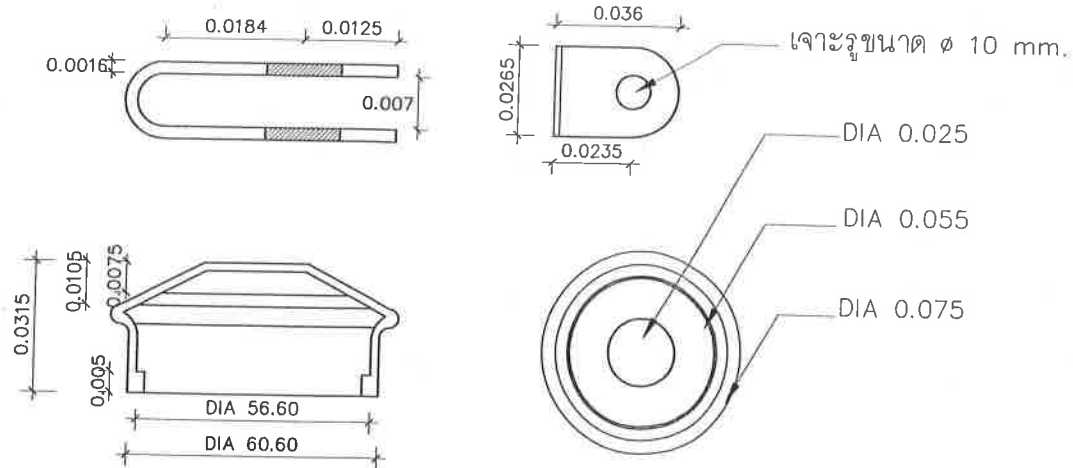
แบบขยาย หัวเสา
