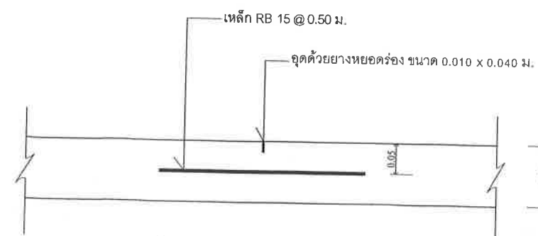
รูปตัด CONTRACTION JOINT SCALE 1 : 100
