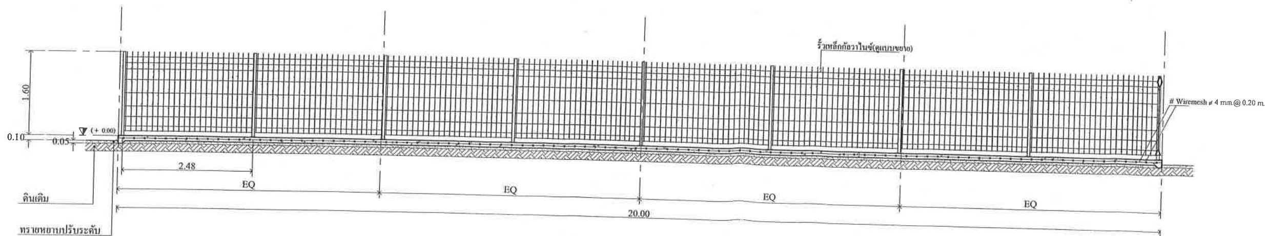
รูปตัด 2 SCALE 1 : 75
