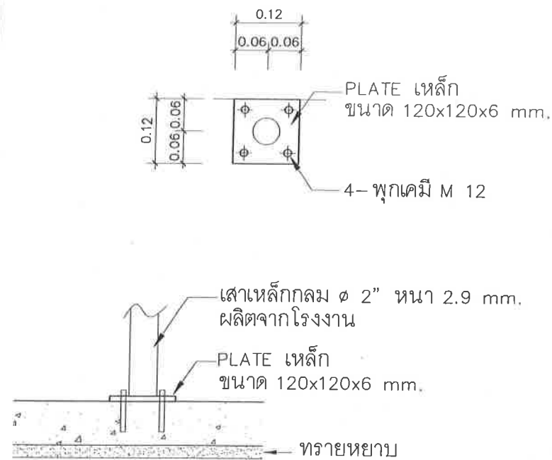
แบบขยาย 1
