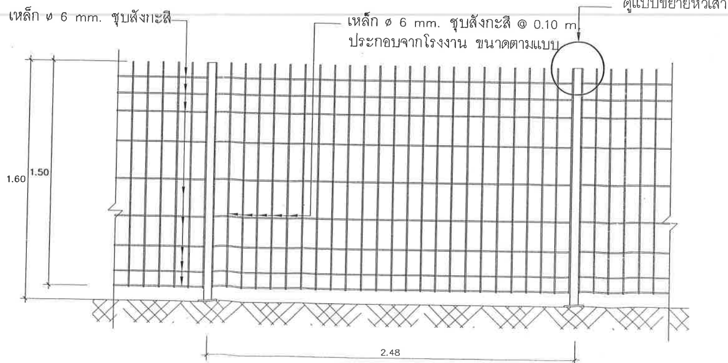
แบบรูปด้านรายละเอียดตัว "LT 1500A"
