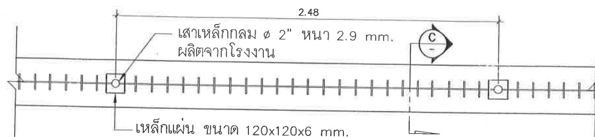
แบบแสดงรายละเอียดตัว "LT 1500A"
