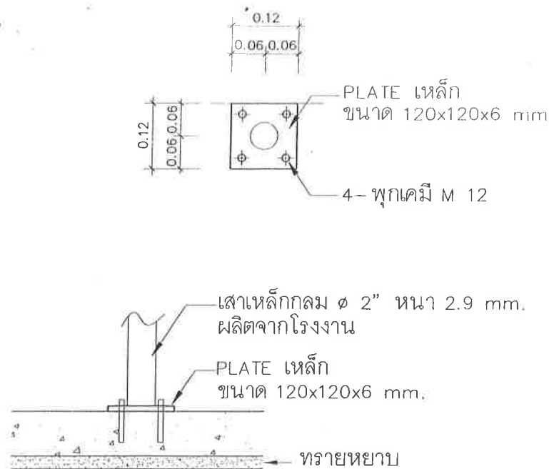
แบบขยาย 1
