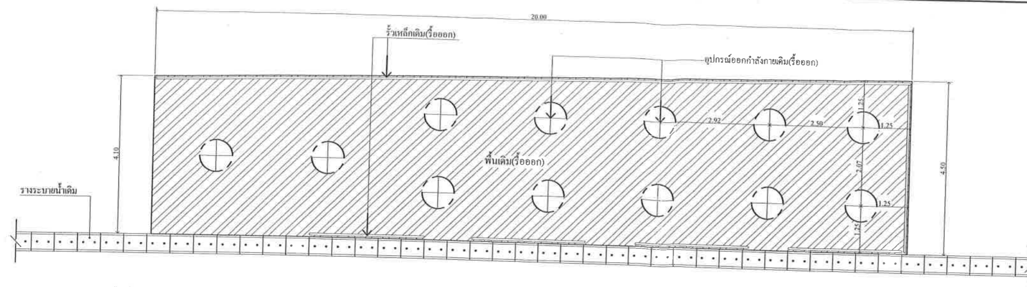
แปลนรื้อถอน SCALE 1:100
