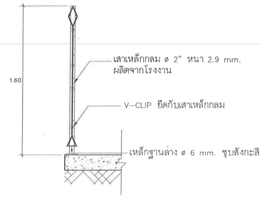
รูปตัด "C" SCALE 1:25
