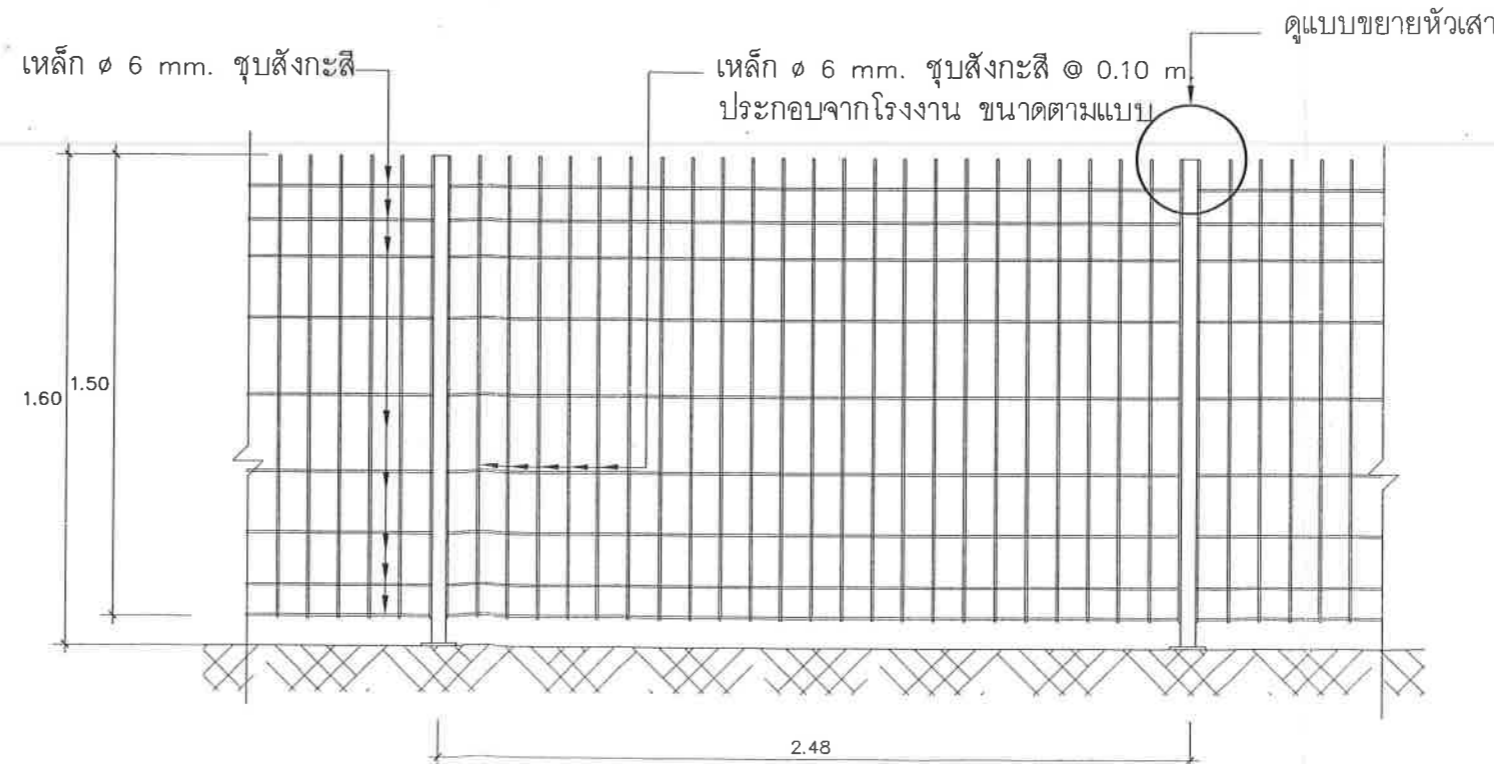
แบบรูปด้านรายละเอียดรั้ว "LT 1500A" SCALE 1:25
