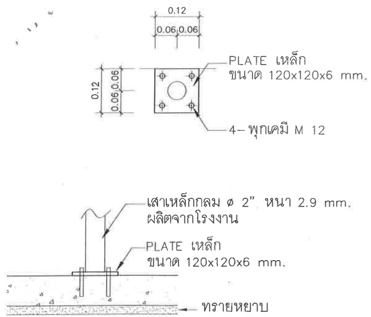
แบบขยาย 1 NOT TO SCALE
