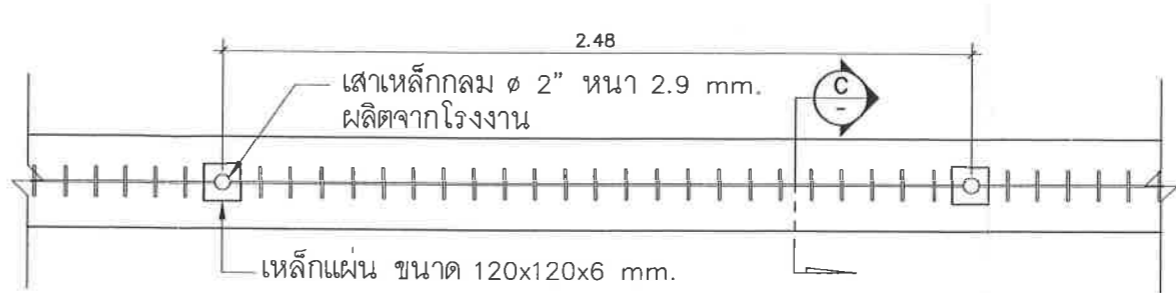
แบบแสดงรายละเอียดรั้ว "LT 1500A" SCALE 1:25
