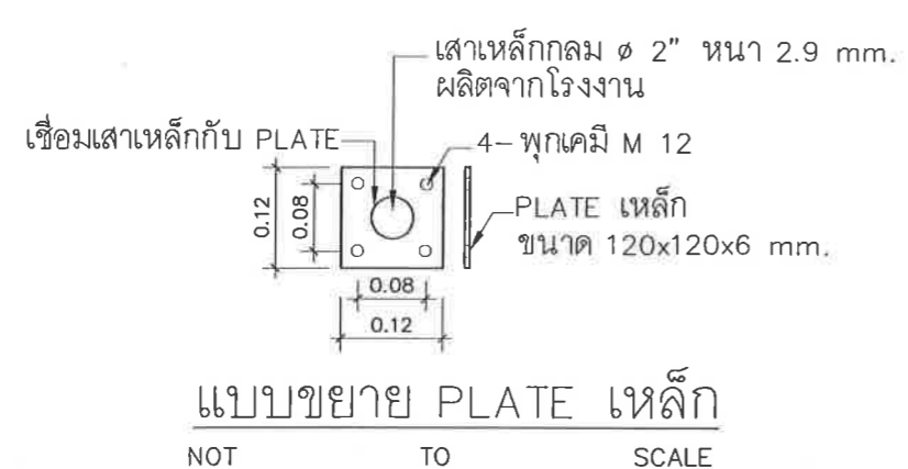
แบบขยาย 1 NOT TO SCALE
