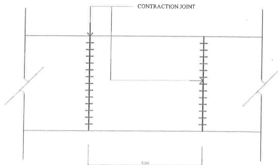
แปลนการวาง CONTRACTION JOINT SCALE 1 : 100
