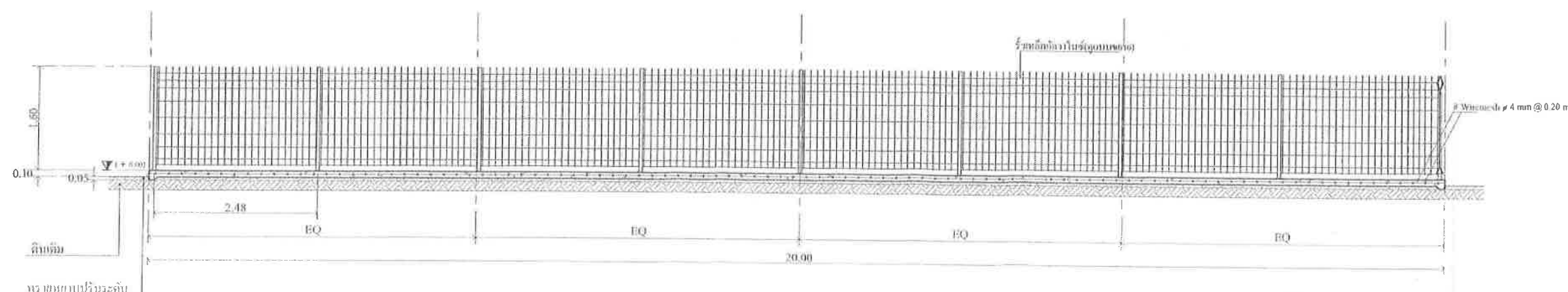
รูปตัด 2 SCALE 1 : 75
