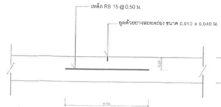
รูปตัด CONTRACTION JOINT SCALE 1 : 100
