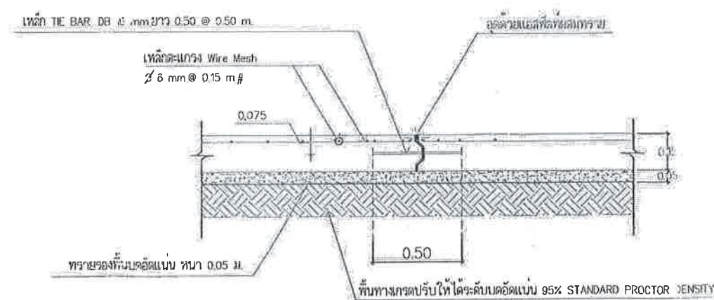
LONGITUDINAL JOINT กึ่งกลางถนนตลอดความยาว
