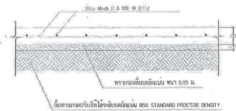
แบบขยายถนน ค.ส.ล.
