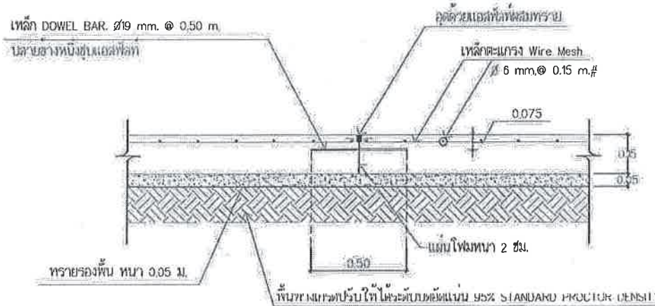
EXPANSION JOINT ทุกความยาวไม่เกิน 30 ม.
