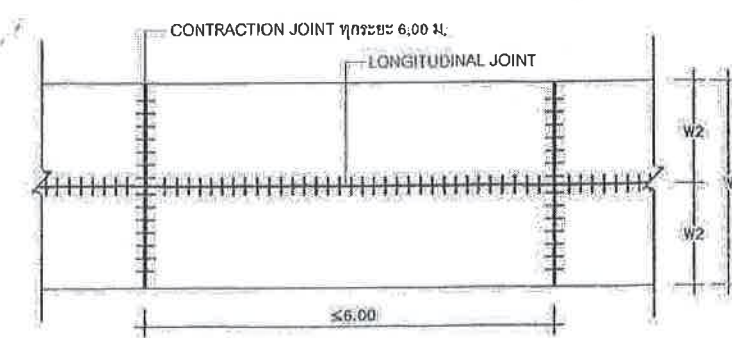
แปลนการวาง CONTRACTION JOINT และ LONGITUDINAL JOINT
