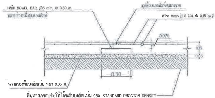
CONTRACTION JOINT ทุกความยาวไม่เกิน 6 ม.
