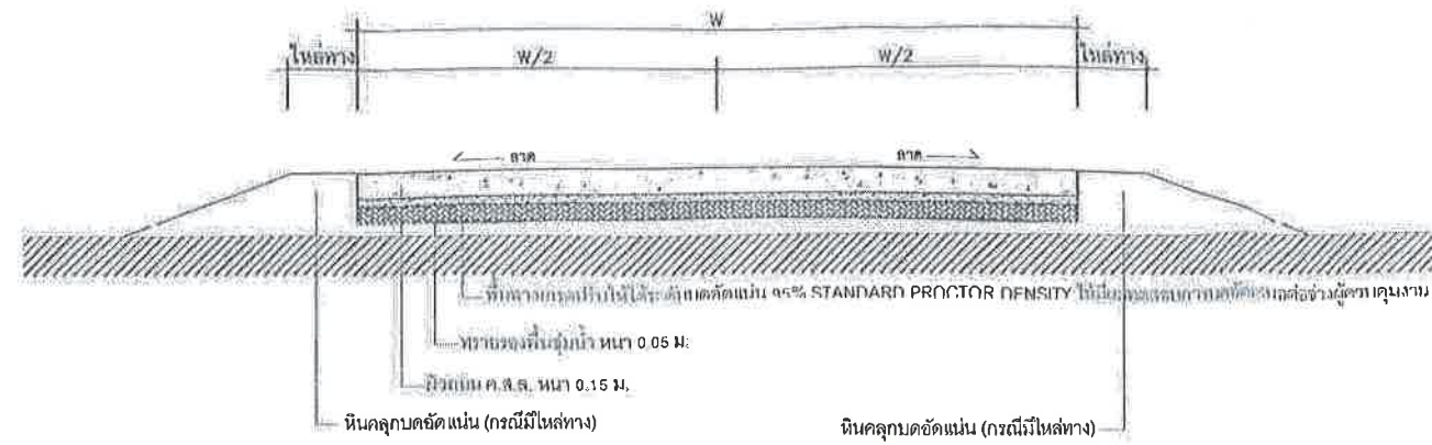
รูปตัดขยายถนน ค.ส.ล.
