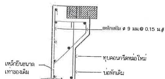
แบบขยายต่อปากบ่อพัก (กรณีที่ 1)
