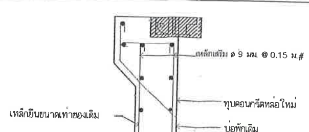
แบบขยายต่อปากบ่อพัก (กรณีที่ 2)
