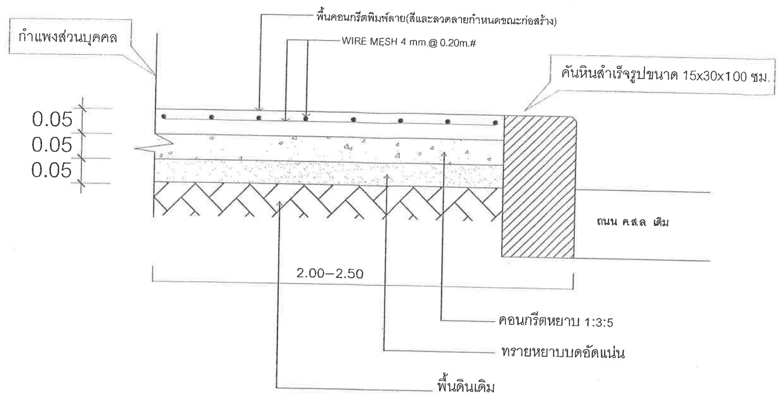
แบบขยายทางเท้า ค.ส.ล. ผิวพิมพ์ลาย NO SCALE
