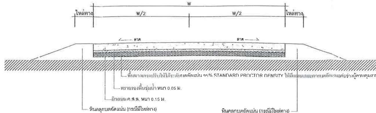
รูปตัดขยายถนน ค.ส.ล.
