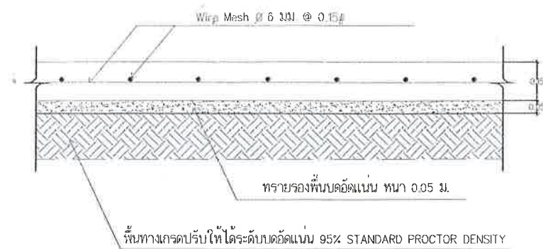
แบบขยายถนน ค.ส.ล. มาตราส่วน No to scale
