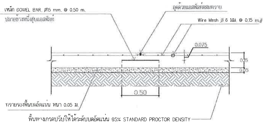
CONTRACTION JOINT ทุกความยาวไม่เกิน 6 ม. มาตราส่วน No to scale
