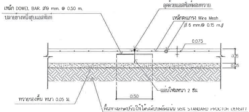
EXPANSION JOINT ทุกความยาวไม่เกิน 30 ม. มาตราส่วน No to scale
