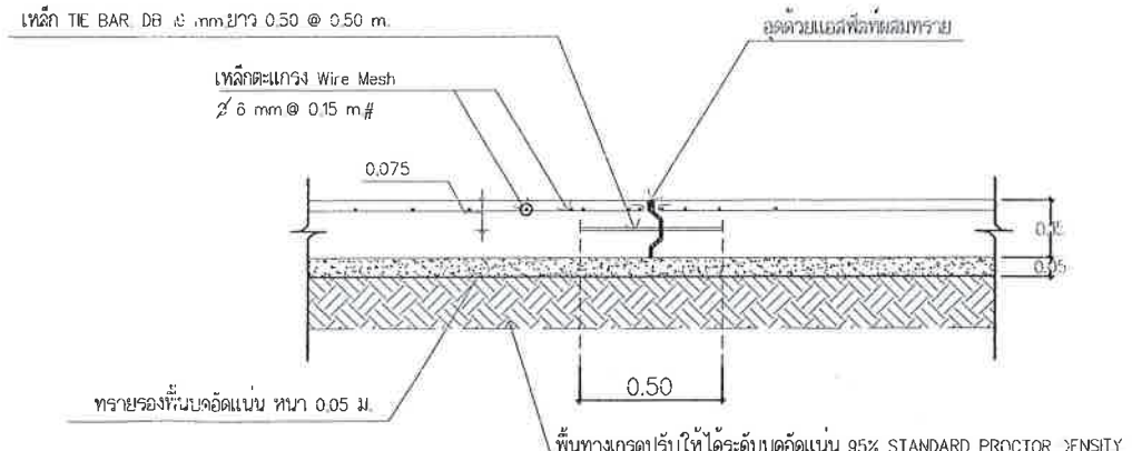
LONGITUDINAL JOINT กึ่งกลางถนนตลอดความยาว มาตราส่วน No to scale
